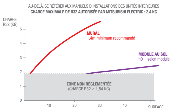
FIGURE B : CHARGES LIMITES INDICATIVES DE R32 SELON EN378 (2016) EN FONCTION DU TYPE D'UNITÉ INTÉRIEURE
