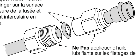
Raccords en acier inoxydable et joint intercalaire en cuivre
