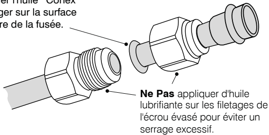
Raccord flare cuivre
