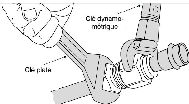
Serrer l'écrou à l'aide d'une clé dynamométrique
